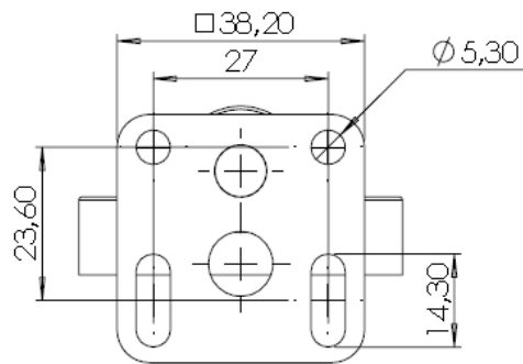
DETAIL B MABSTAB 1 : 1
