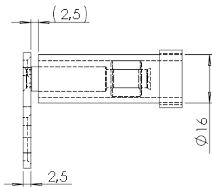
DETAIL A MABSTAB 1 : 1
