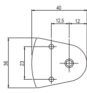
značky pre zarovnanie korpusu
